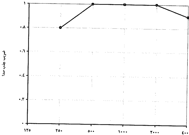
بسامد مرکزی بندهای یکهنگامی به هرتز
