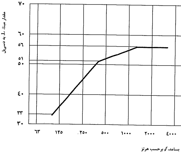
شکل ۱۸-۳-۴: نمودار مقادیر مینا برای صدای هواپرد، در بندهای یک‌سوم هنگامی
